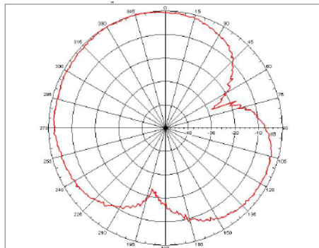
E-PLANE
